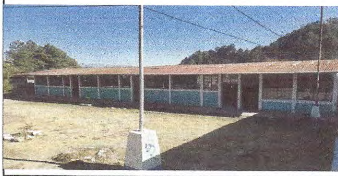
Foto 2: En la se observa la lámina del techo que será sustituido por lámina troquelada aluzinc calibre 26 que será de 306.99 mts cuadrados
